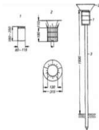
Слика 24. Изглед Bergerhoff колектора
