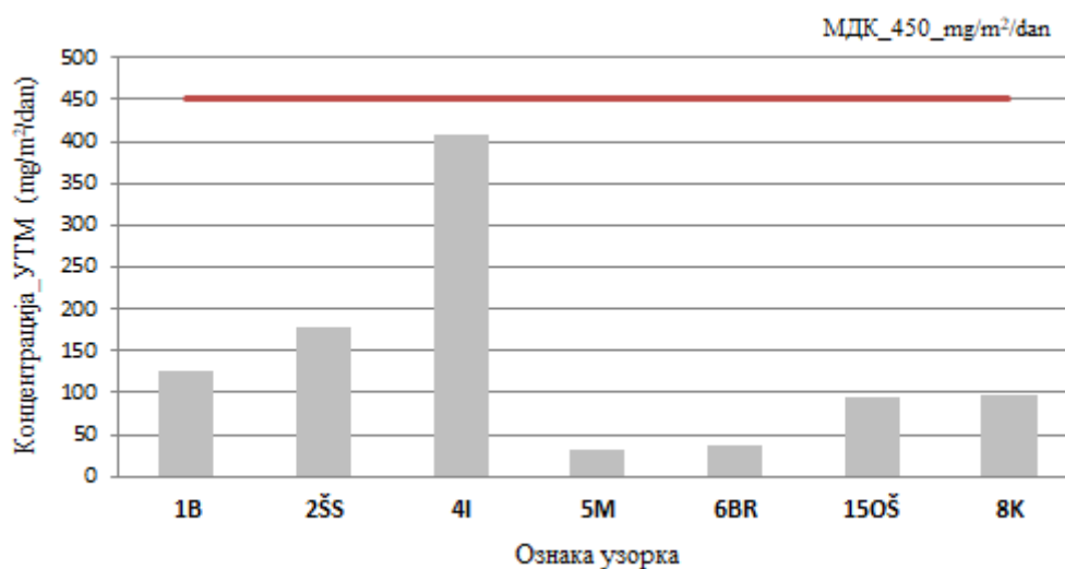
Слика 35. Резултати концентрације УТМ, на 7 мерних места, за октобар 2021.
