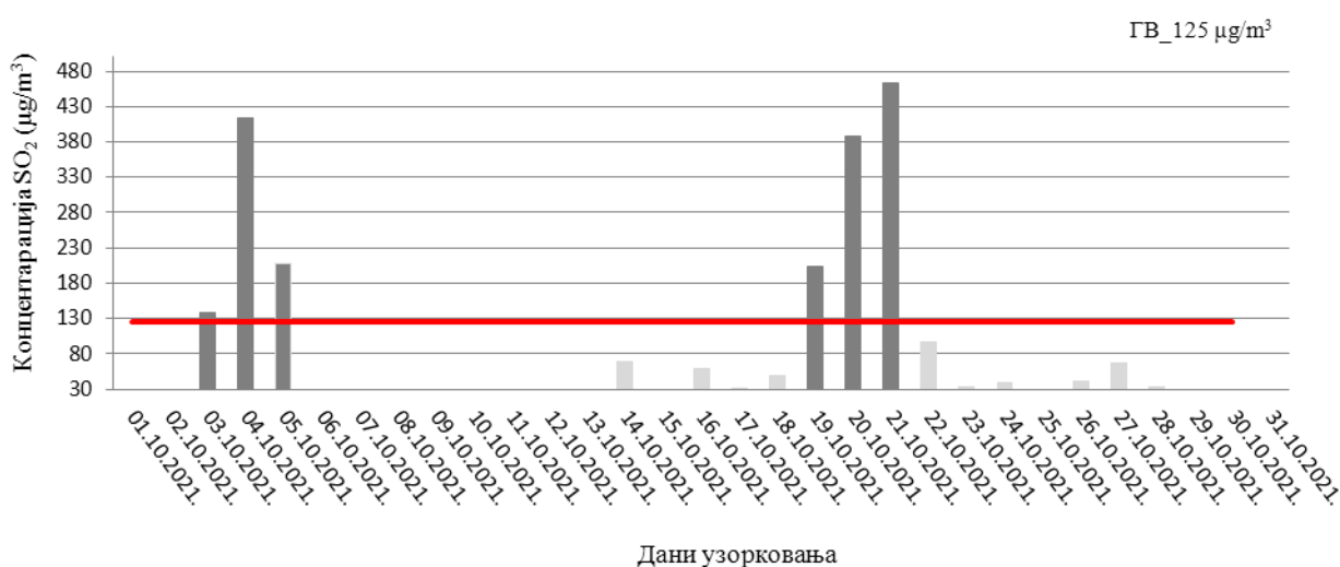
Слика 25. Резултати концентрације SO_2 у ваздуху, на мерном месту 47755-21 JP Југопетрол
