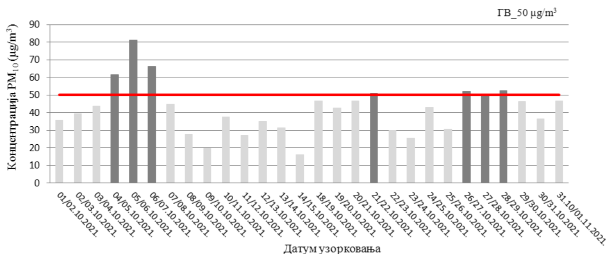
Слика 31. Резултати концентрације PM_{10} у ваздуху, на мерном месту 47755-21_ОШ_Оштрељ
