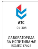
Табела 5. Приказ вредности концентрација суспендованих честица PM_{10} и матала у PM_{10} , за месец октобар 2021, на мерном месту 47755-21_ОШ_Оштрелј
