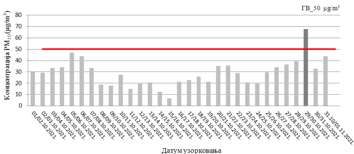
Слика 29. Резултати концентрације PM_{10} у ваздуху, на мерном месту 47755-21_K_Кривељ
