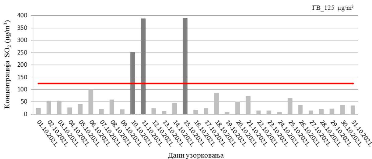
Слика 27. Резултати концентрације SO_2 у ваздуху, на мерном месту 47755-21_П_Градски парк
