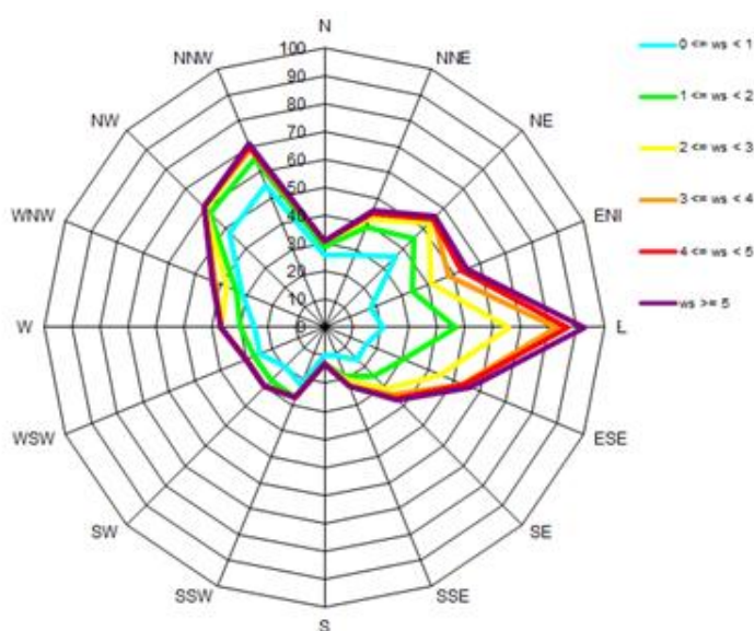
Слика 4. Графички приказ руже ветра, за период од 01.10 до 31.10.2021.
