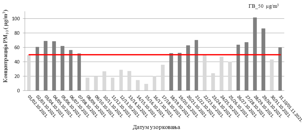
Слика 32. Резултати концентрације PM_{10} у ваздуху, на мерном месту 47755-21_Вз_Брезоник
