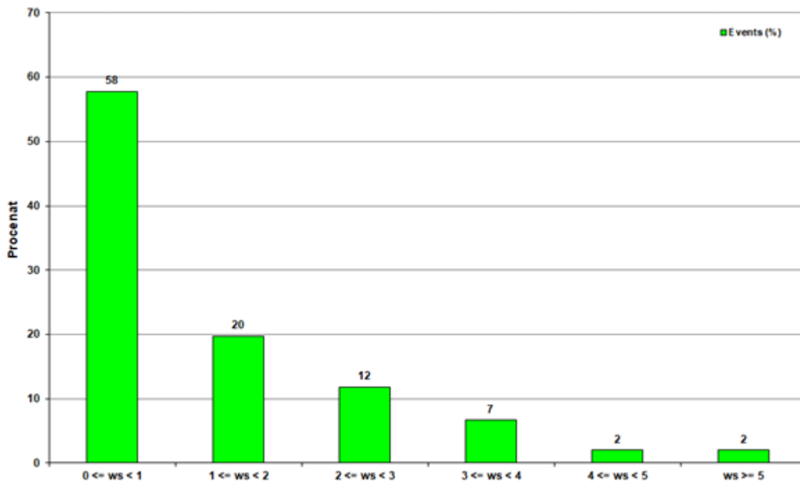
Слика 7. Графички приказ расподеле класа брзина ветра, за период од 01.10 до 31.10.2021.
