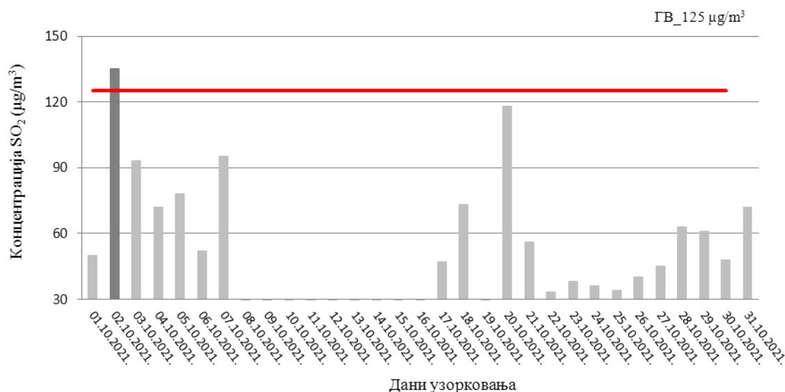
Слика 26. Резултати концентрације SO_2 у ваздуху, на мерном месту 47755-21 F Технички факултет
