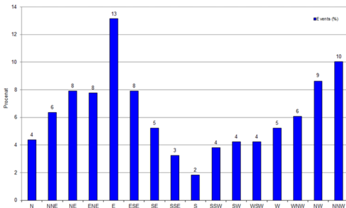
Слика 6. Графички приказ расподеле праваца ветра, за период од 01.10 до 31.10.2021.
