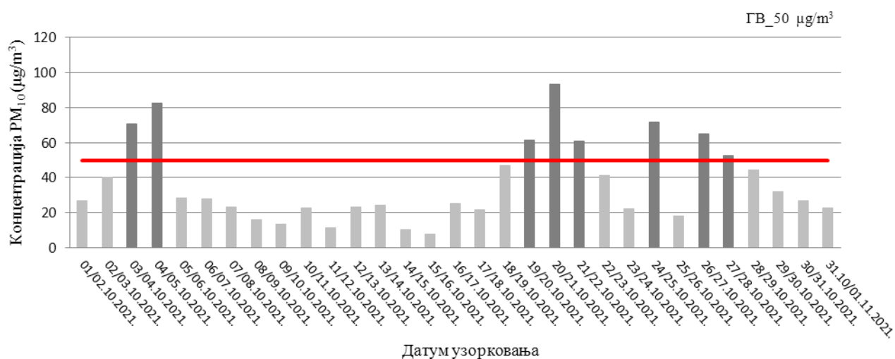
Слика 30. Резултати концентрације PM_{10} у ваздуху, на мерном месту 47755-21_JP_Југопетрол
