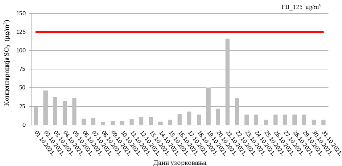
Слика 28. Резултати концентрације SO_2 у ваздуху, на мерном месту 47755-21_И_Институт
