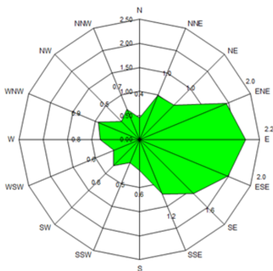
Слика 5. Графички приказ средње брзине ветра из појединих праваца, за период од 01.10 до 31.10.2021.
