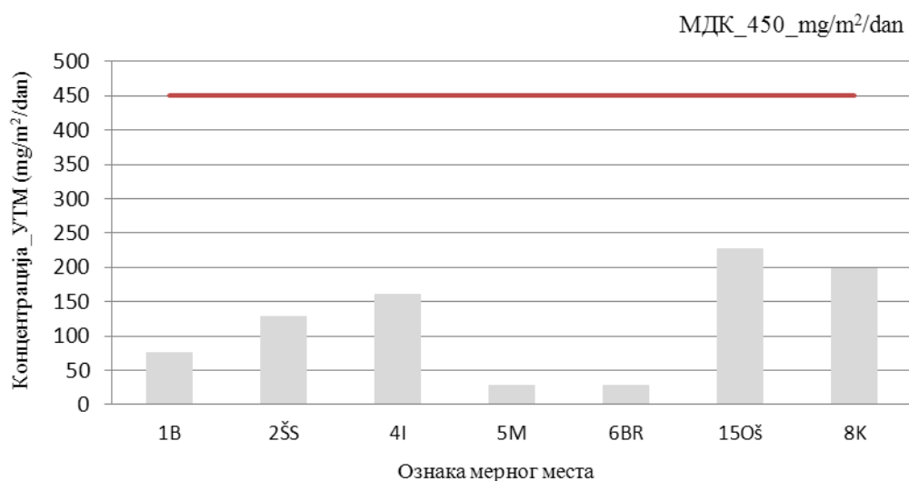
Слика 34. Резултати концентрације УТМ, на 7 мерних места, за месец март 2021.
