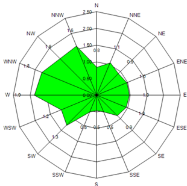
Слика 5. Графички приказ средње брзине ветра из појединих праваца, за период од 01.03. до 31.03.2021.
