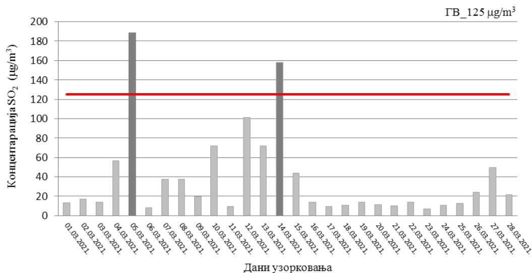
Слика 27. Резултати концентрације SO_2 у ваздуху, на мерном месту 44889-21_I_Институт
