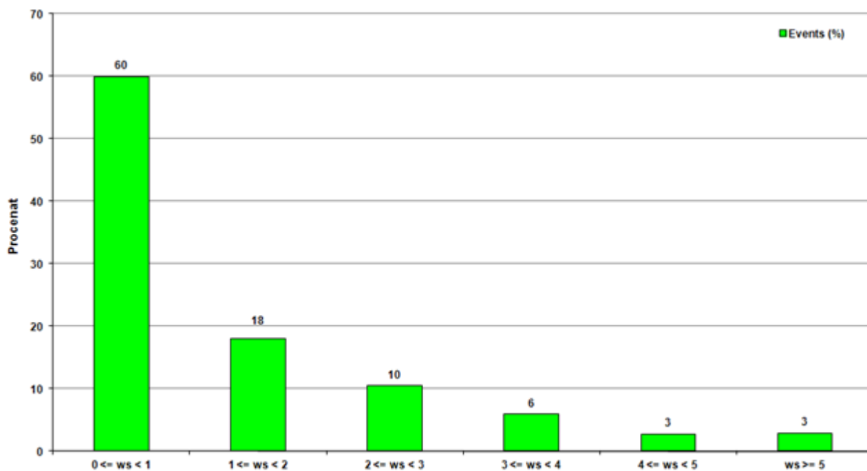
Слика 7. Графички приказ расподеле класа брзина ветра, за период од 01.03. до 31.03.2021.
