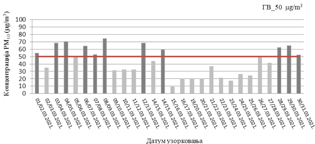
Слика 30. Резултати концентрације PM_{10} у ваздуху, на мерном месту 44889-21_ОШ_Оштрељ
