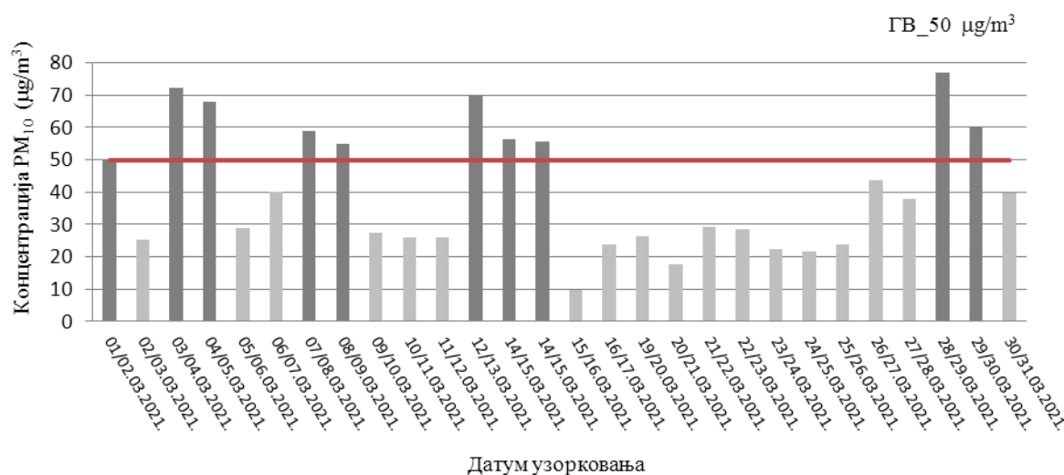
Слика 31. Резултати концентрације PM_{10} у ваздуху, на мерном месту 44889-21_Вз_Брезоник
