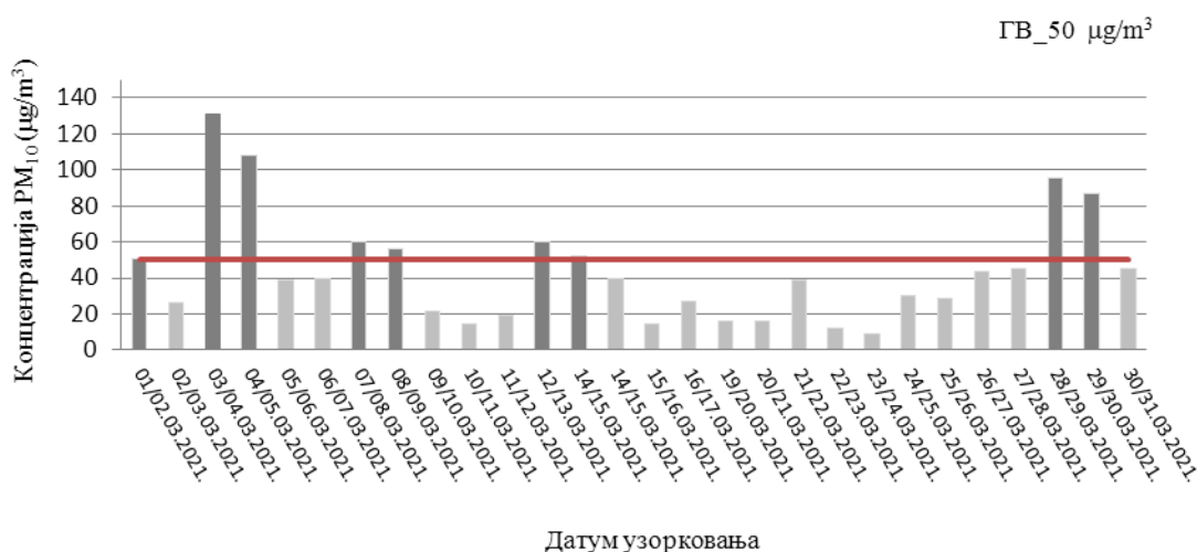
Слика 29. Резултати концентрације PM_{10} у ваздуху, на мерном месту 44889-21_ЈП_Југопетрол
