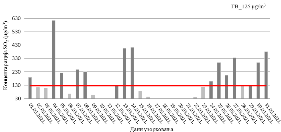
Слика 24. Резултати концентрације SO_2 у ваздуху, на мерном месту 44889-21_JP_Југопетрол
