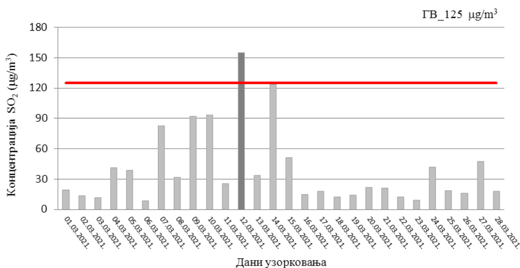
Слика 26. Резултати концентрације SO_2 у ваздуху, на мерном месту 44889-21_P_Градски парк
