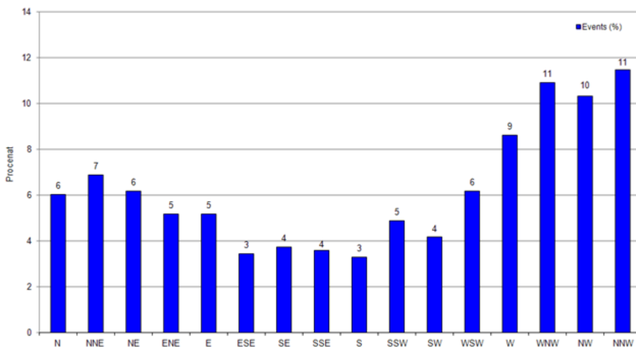
Слика 6. Графички приказ расподеле праваца ветра, за период од 01.03. до 31.03.2021.
