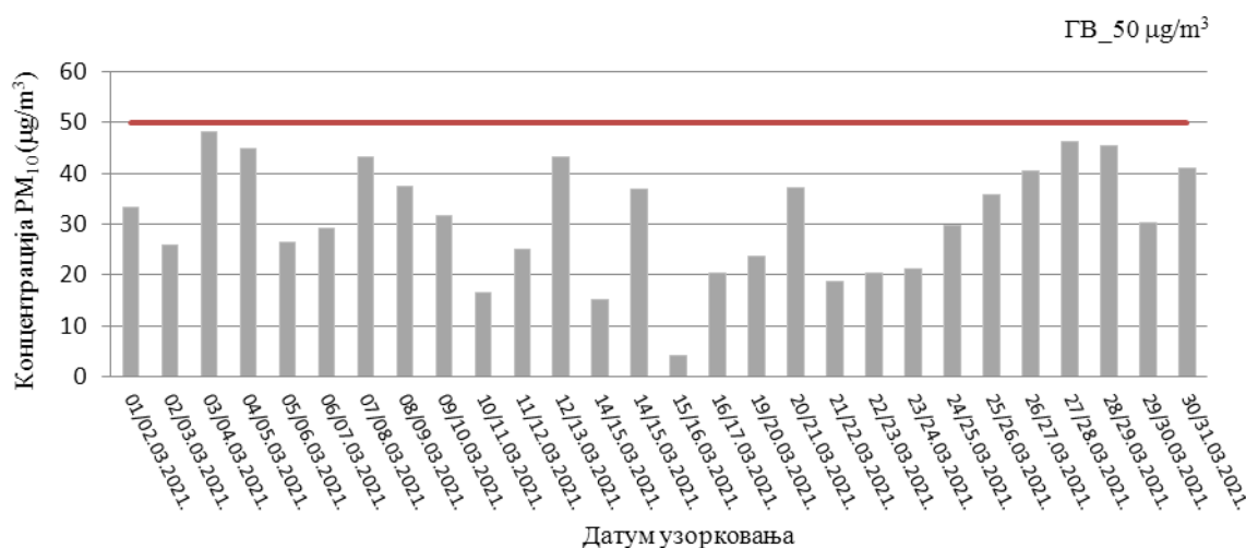
Слика 28. Резултати концентрације PM_{10} у ваздуху, на мерном месту 44889-21_К_Кривељ
