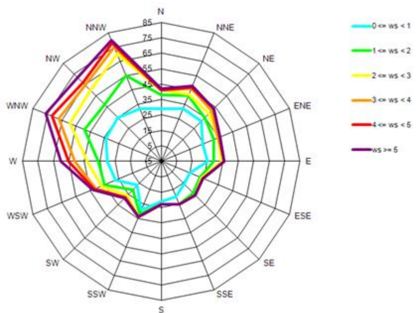
Слика 4. Графички приказ руже ветра, за период од 01.03. до 31.03.2021.
