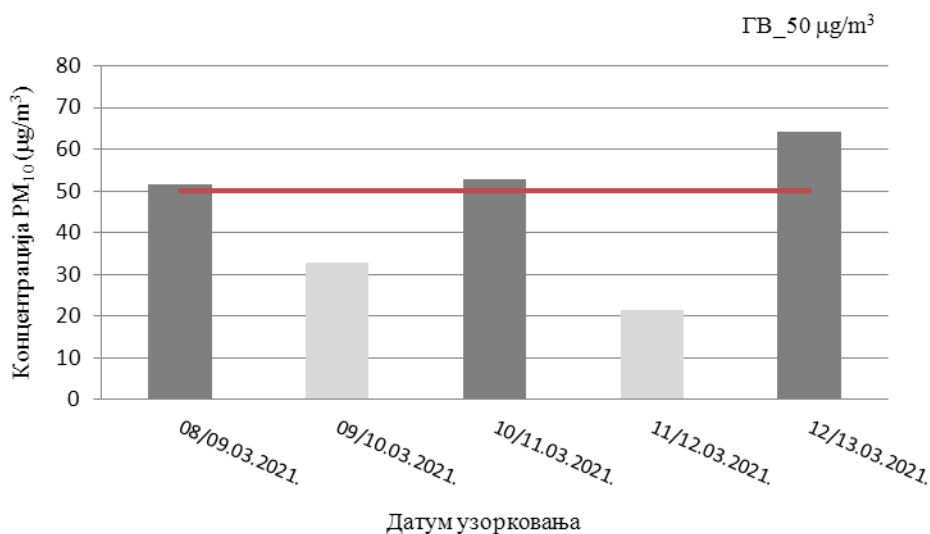
Слика 32. Резултати концентрације PM_{10} у ваздуху, на мерном месту 44889-21_I_Институт
