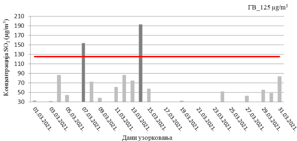
Слика 25. Резултати концентрације SO_2 у ваздуху, на мерном месту 44889-21_F_Технички факултет
