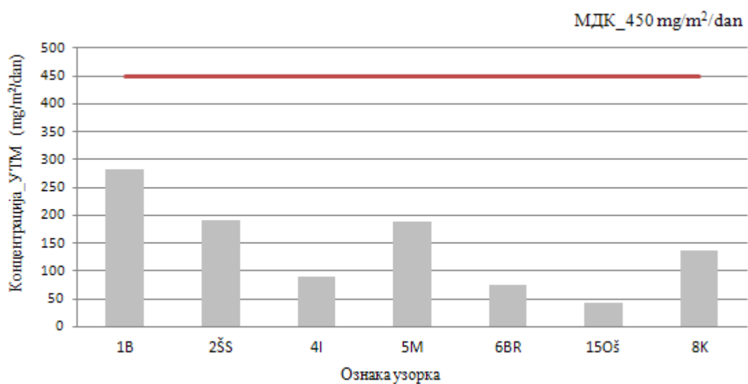
Слика 34. Резултати концентрације УТМ, на 7 мерних места, за мај 2021.
