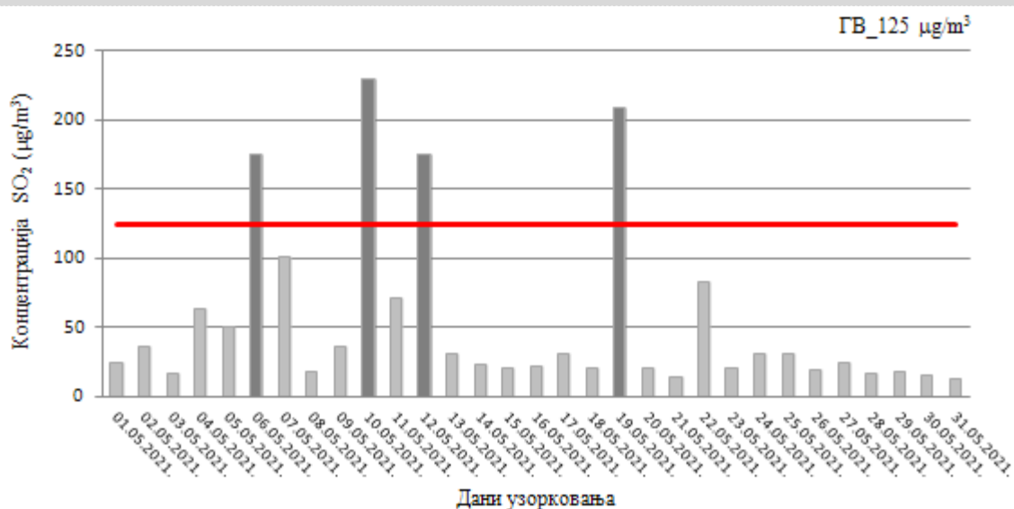
Слика 26. Резултати концентрације SO_2 у ваздуху, на мерном месту 45404-21_P Градски парк
