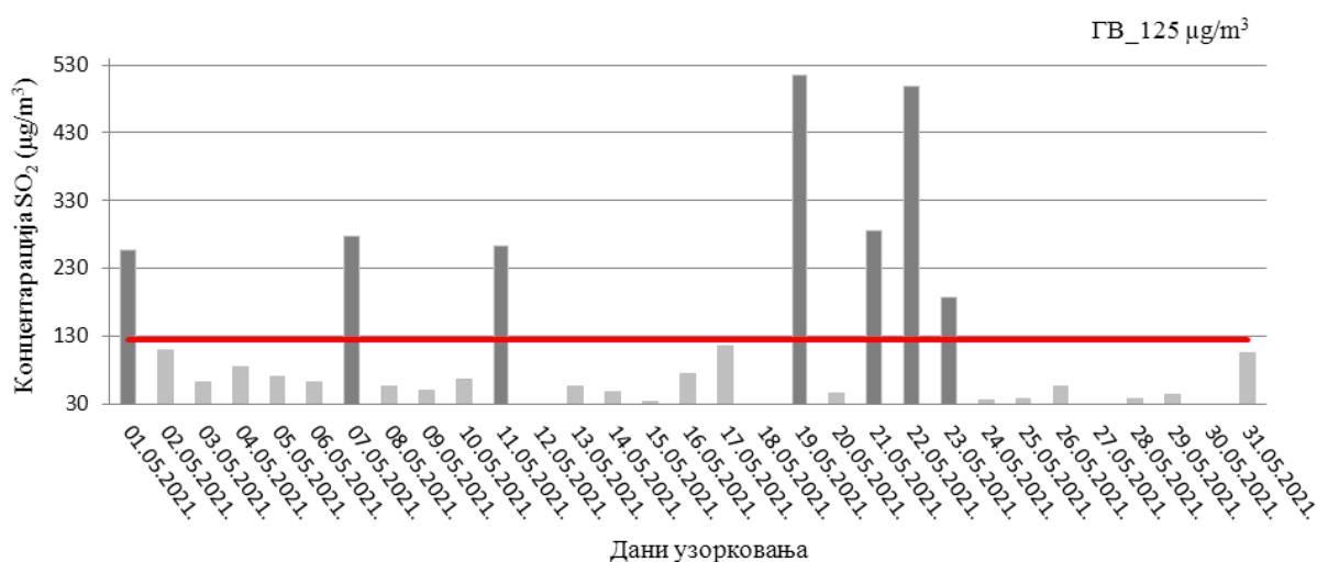
Слика 24. Резултати концентрације SO_2 у ваздуху, на мерном месту 45404-21_JP_Југопетрол
