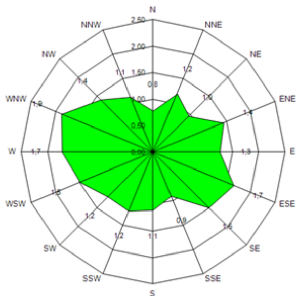
Слика 5. Графички приказ средње брзине ветра из појединих праваца, за период од 01.05. до 31.05.2021.
