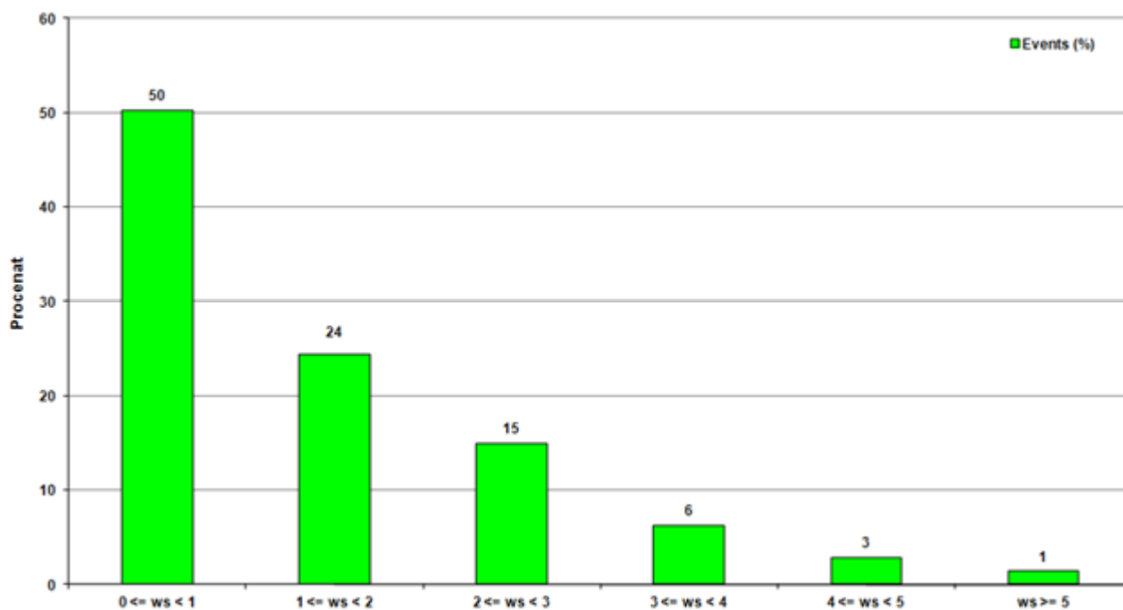
Слика 7. Графички приказ расподеле класа брзина ветра, за период од 01.05. до 31.05.2021.
