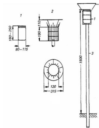
Слика 25. Изглед Bergerhoff колектора
