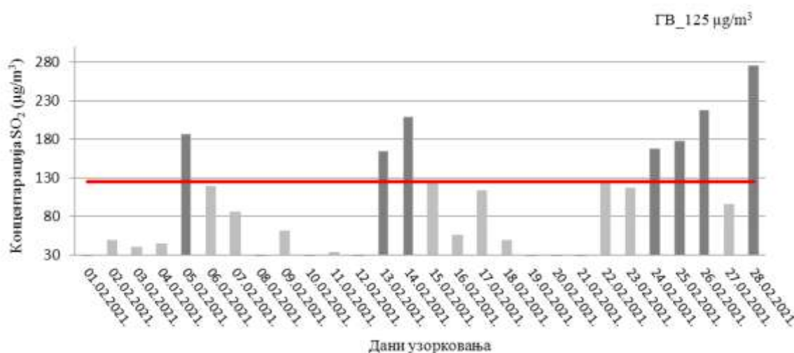
Слика 24. Резултати концентрације SO_2 у ваздуху, на мерном месту 44290-21_JP_Југопетрол
