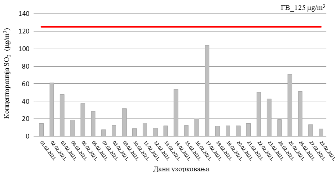
Слика 27. Резултати концентрације SO_2 у ваздуху, на мерном месту 44290-21_I_Институт
