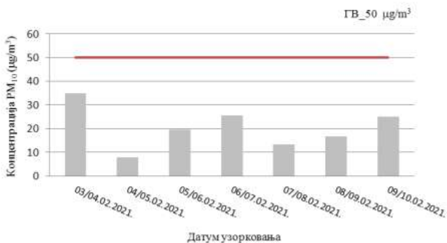
Слика 33. Резултати концентрације PM_{10} у ваздуху, на мерном месту 43752-21_P_Градски парк
