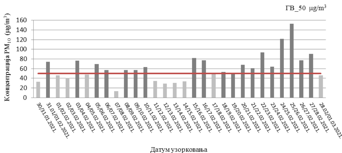
Слика 31. Резултати концентрације PM_{10} у ваздуху, на мерном месту 44290-21_Вз_Брезоник
