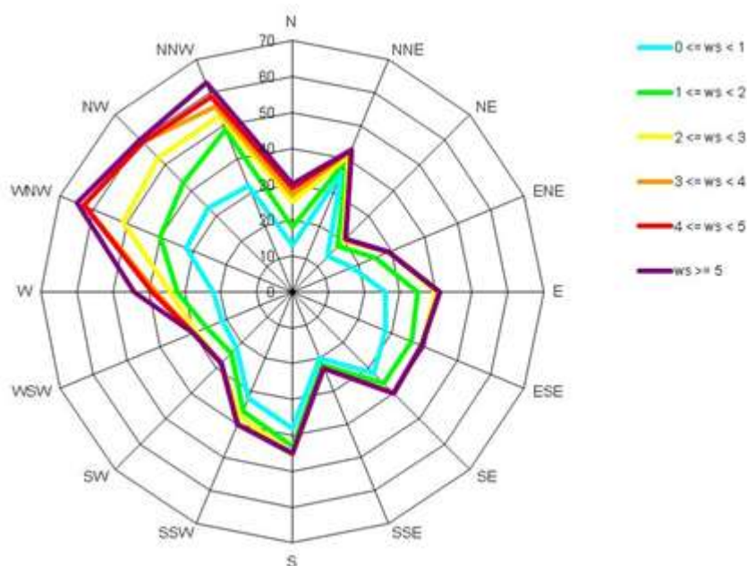
Слика 4. Графички приказ руже ветра, за период од 01.02. до 28.02.2021.
