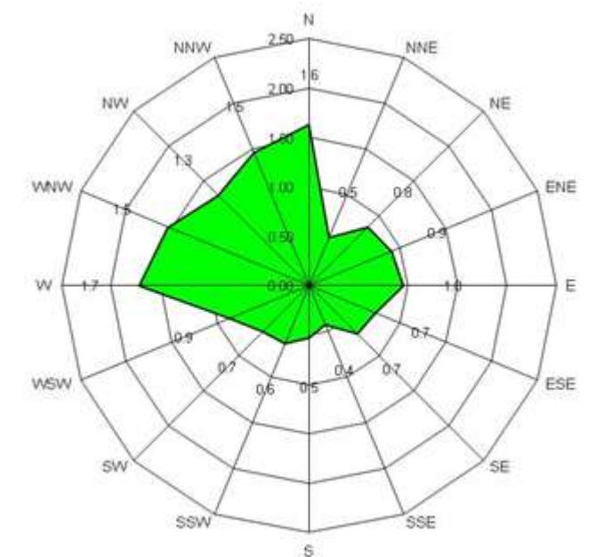
Слика 5. Графички приказ средње брзине ветра из појединих праваца, за период од 01.02. до 28.02.2021.
