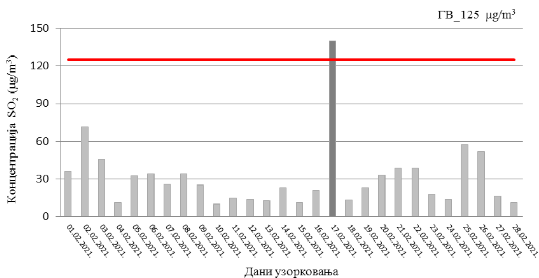
Слика 26. Резултати концентрације SO_2 у ваздуху, на мерном месту 44290-21_P_Градски парк
