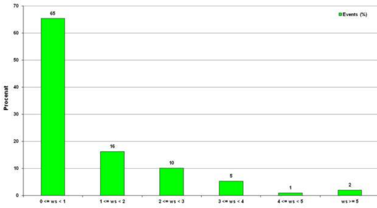
Слика 7. Графички приказ расподеле класа брзина ветра, за период од 01.02. до 28.02.2021.
