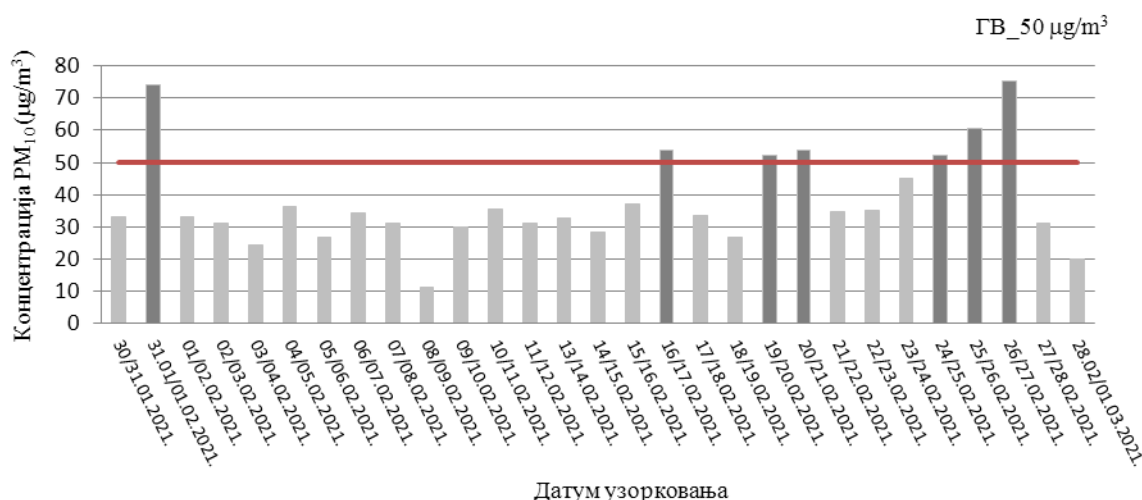
Слика 28. Резултати концентрације PM_{10} у ваздуху, на мерном месту 44290-21_К_Кривељ
