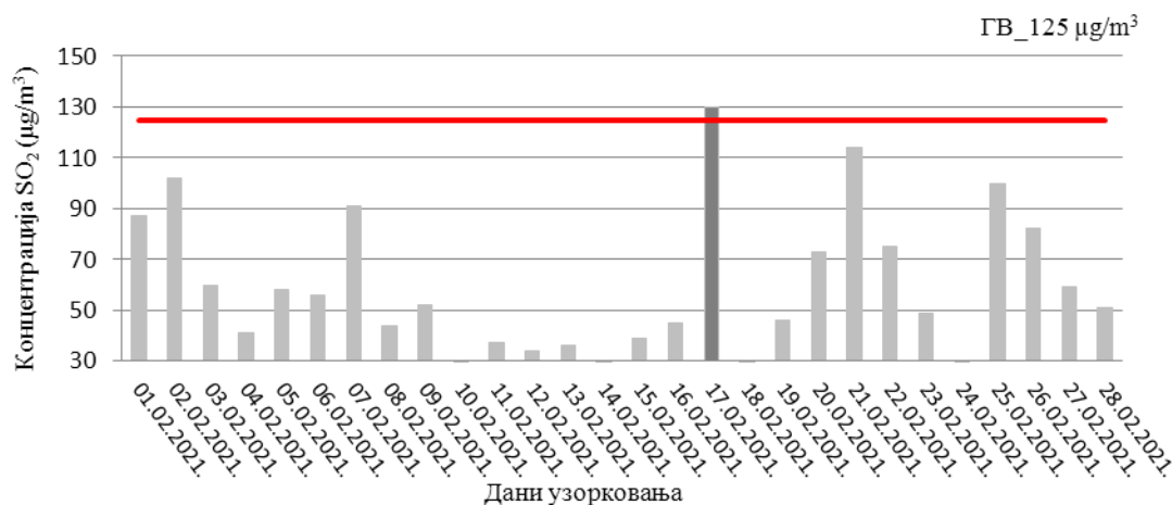
Слика 25. Резултати концентрације SO_2 у ваздуху, на мерном месту 44290-21_F_Технички факултет
