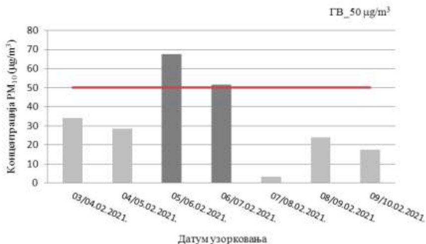
Слика 32. Резултати концентрације PM_{10} у ваздуху, на мерном месту 44290-21_I_Институт
