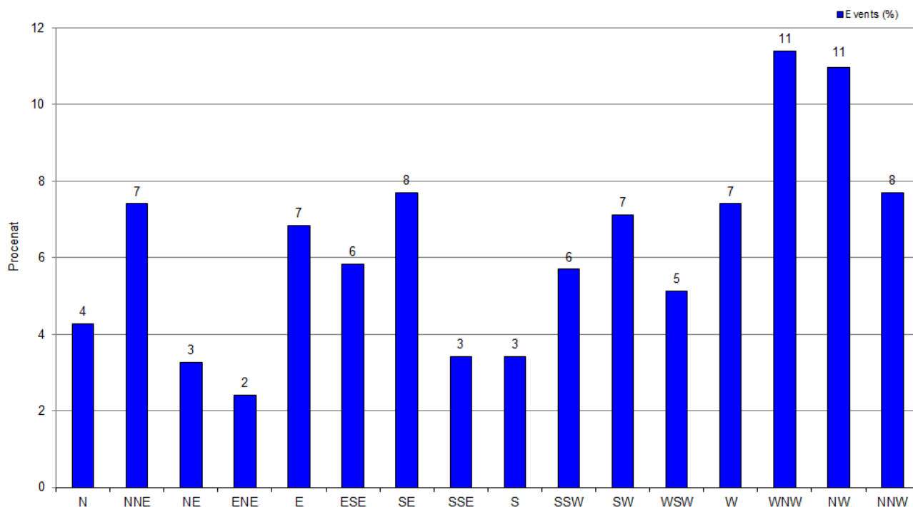
Слика 6. Графички приказ расподеле праваца ветра, за период од 01.12 до 31.12.2021.
