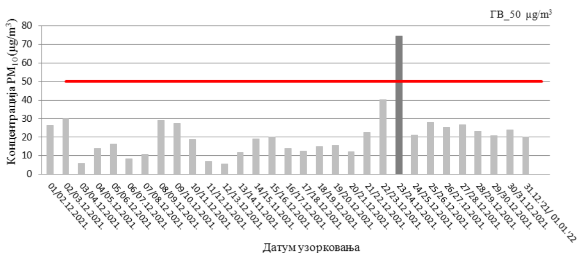
Слика 29. Резултати концентрације PM_{10} у ваздуху, на мерном месту 48468-21_К_Кривељ
