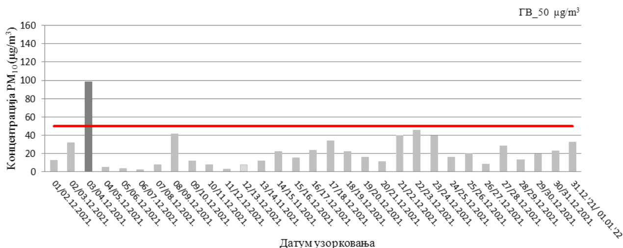
Слика 30. Резултати концентрације PM_{10} у ваздуху, на мерном месту 48468-21_ЈП_Југопетрол
