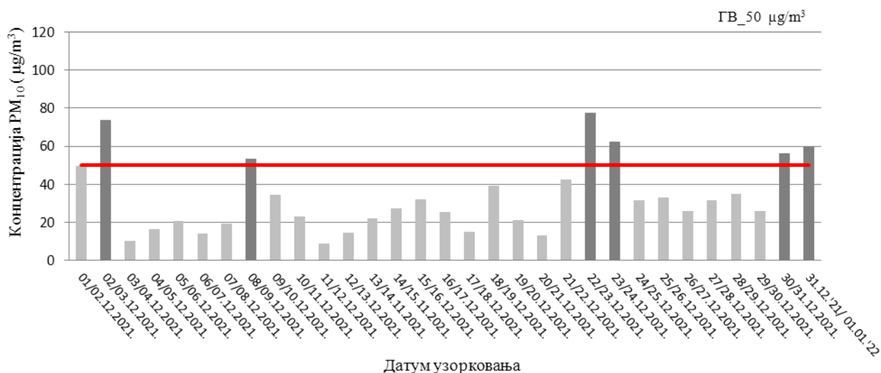
Слика 32. Резултати концентрације PM_{10} у ваздуху, на мерном месту 48468-21_Вз_Брезоник
