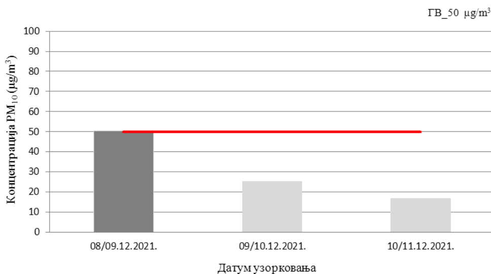
Слика 33. Резултати концентрације PM_{10} у ваздуху, на мерном месту 48468-21_I_Институт
