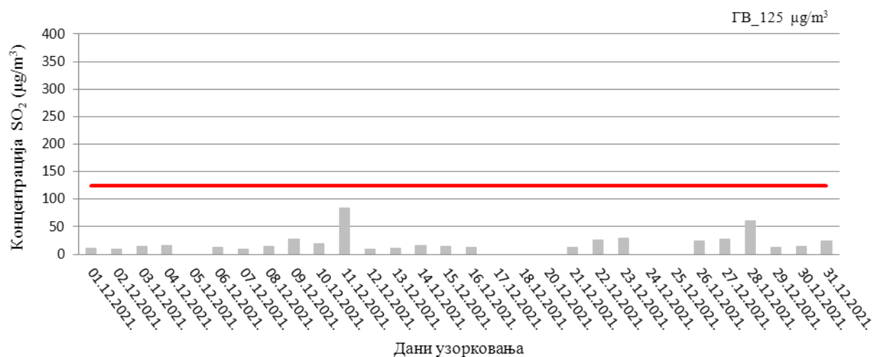
Слика 27. Резултати концентрације SO_2 у ваздуху, на мерном месту 48468-21_P Градски парк
