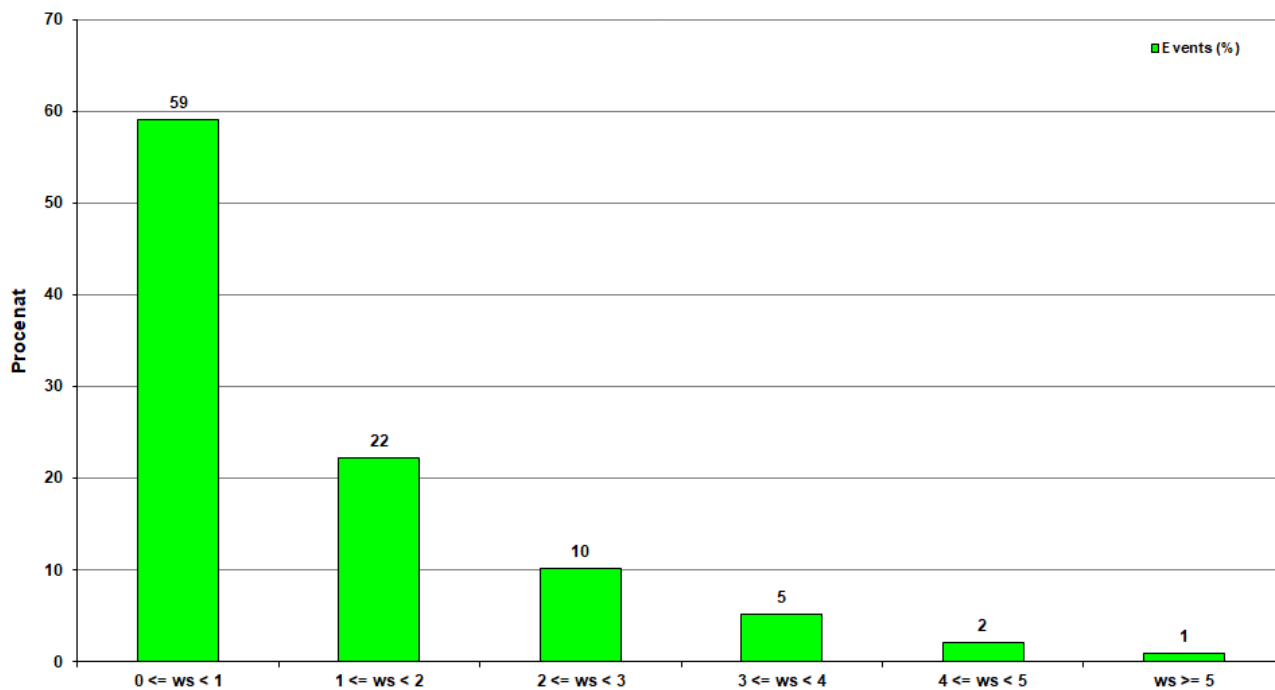
Слика 7. Графички приказ расподеле класа брзина ветра, за период од 01.12 до 31.12.2021.
