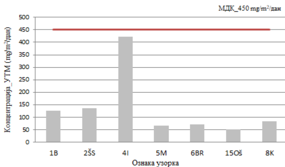
Слика 35. Резултати концентрације УТМ, на 7 мерних места, за децембар 2021.
