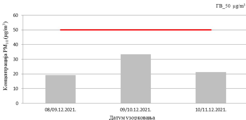
Слика 34. Резултати концентрације PM_{10} у ваздуху, на мерном месту 48468-21_P_Градски парк
