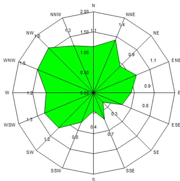
Слика 5. Графички приказ средње брзине ветра из појединих праваца, за период од 01.12 до 31.12.2021.
