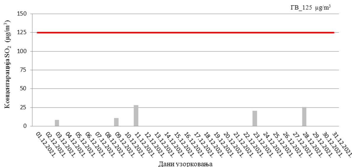
Слика 28. Резултати концентрације SO_2 у ваздуху, на мерном месту 48468-21_I Институт
