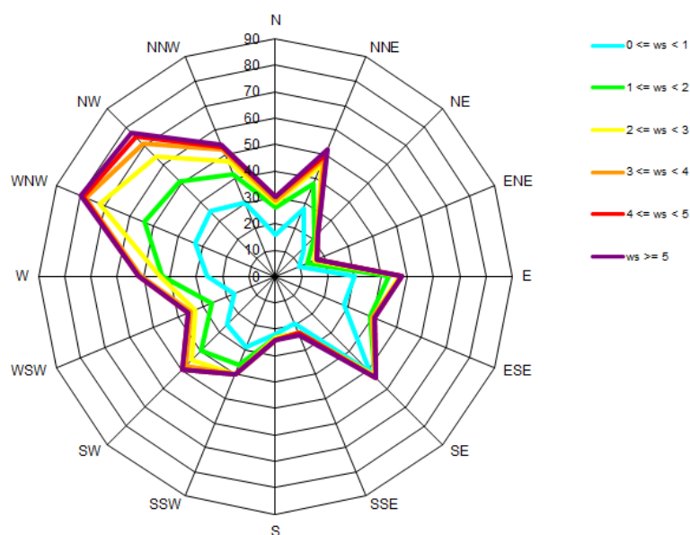
Слика 4. Графички приказ руже ветра, за период од 01.12 до 31.12.2021.
