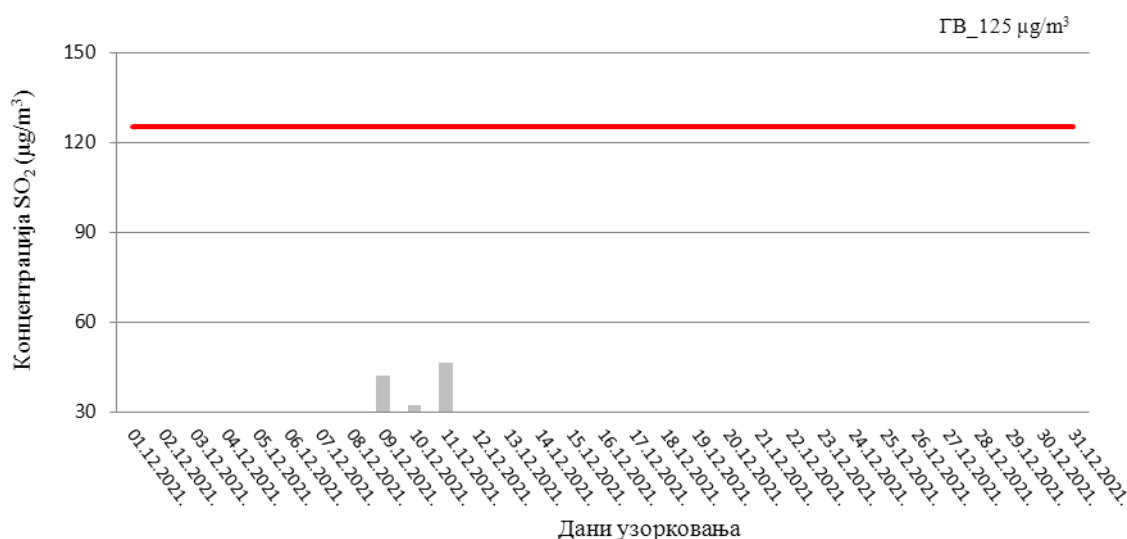
Слика 26. Резултати концентрације SO_2 у ваздуху, на мерном месту 48468-21_F_Технички факултет
