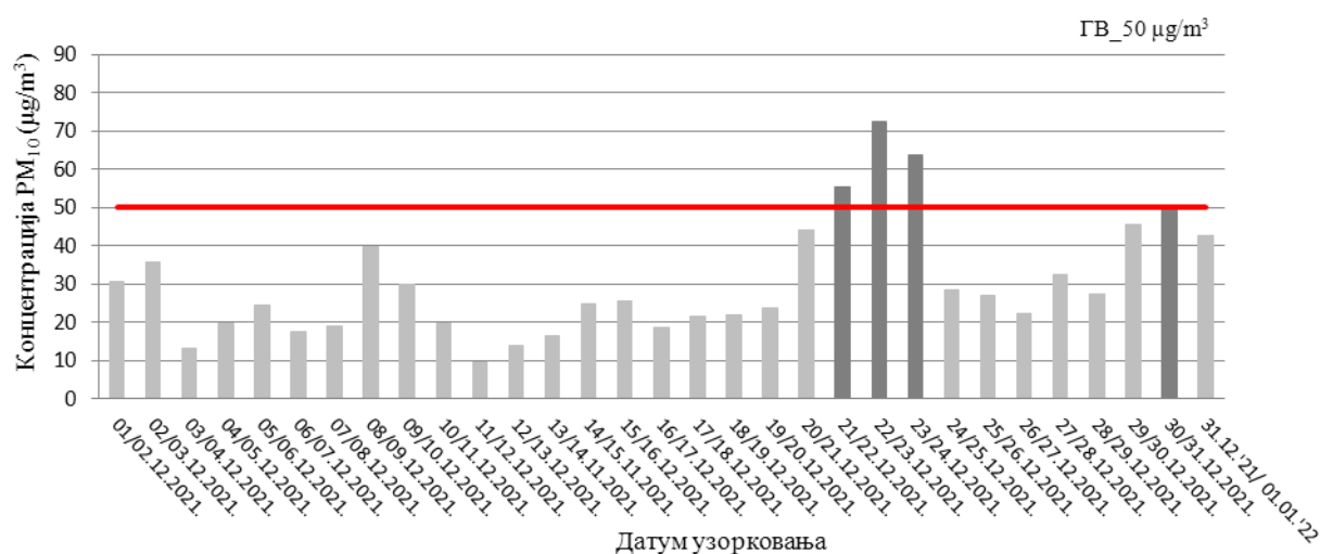
Слика 31. Резултати концентрације PM_{10} у ваздуху, на мерном месту 48468-21_ОШ_Оштрељ
