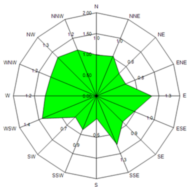
Слика 5. Графички приказ средње брзине ветра из појединих праваца, за период од 01.08. до 31.08.2021.
