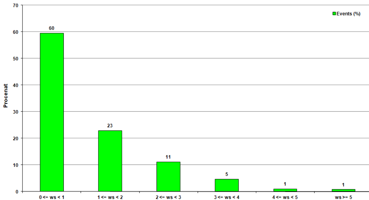
Слика 7. Графички приказ расподеле класа брзина ветра, за период од 01.08. до 31.08.2021.
