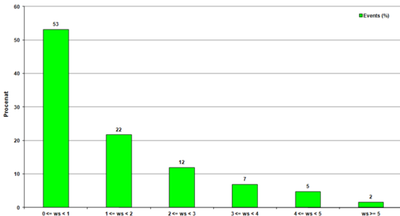
Слика 7. Графички приказ расподеле класа брзина ветра, за период од 01.04. до 30.04.2021.
