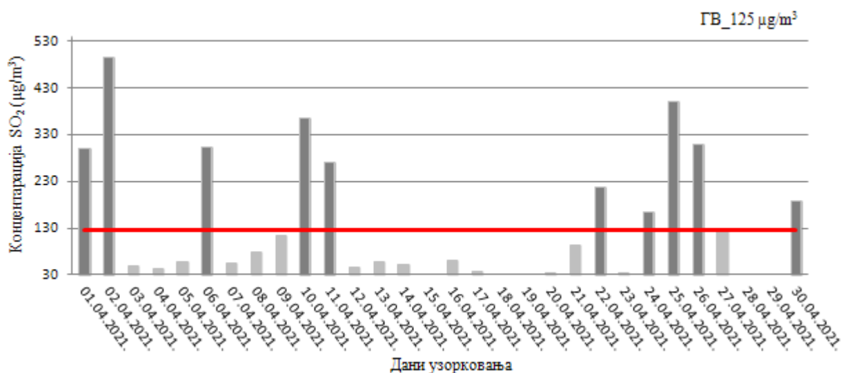
Слика 24. Резултати концентрације SO_2 у ваздуху, на мерном месту 44899-21_JP_Југопетрол
