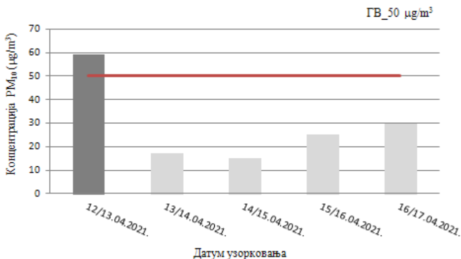
Слика 32. Резултати концентрације PM_{10} у ваздуху, на мерном месту 44899-21_I_Институт
