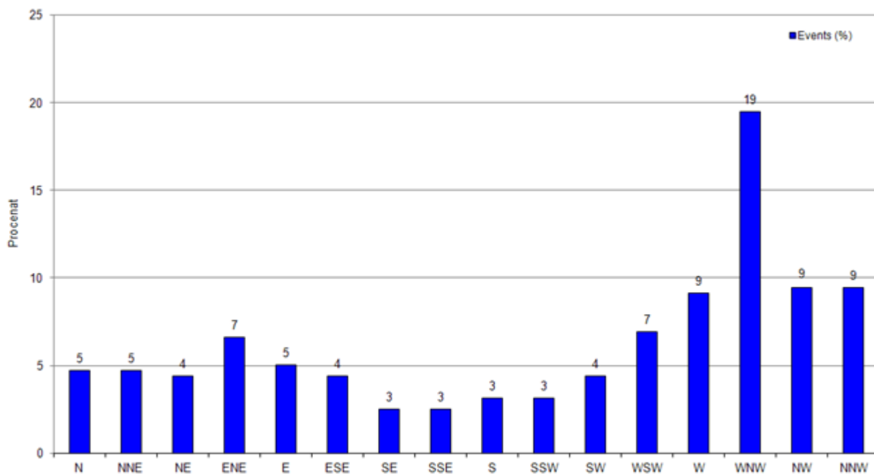
Слика 6. Графички приказ расподеле праваца ветра, за период од 01.04. до 30.04.2021.
