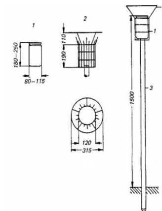
Слика 23. Изглед Bergerhoff колектора
