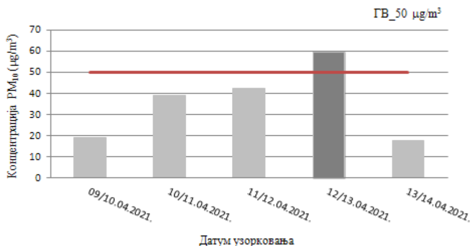
Слика 33. Резултати концентрације PM_{10} у ваздуху, на мерном месту 44899-21_P_Градски парк
