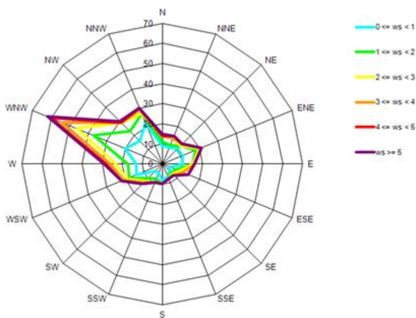
Слика 4. Графички приказ руже ветра, за период од 01.04. до 30.04.2021.
