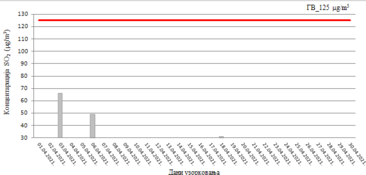
Слика 27. Резултати концентрације SO_2 у ваздуху, на мерном месту 44899-21_I Институт
