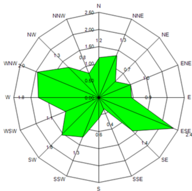
Слика 5. Графички приказ средње брзине ветра из појединих праваца, за период од 01.04. до 30.04.2021.
