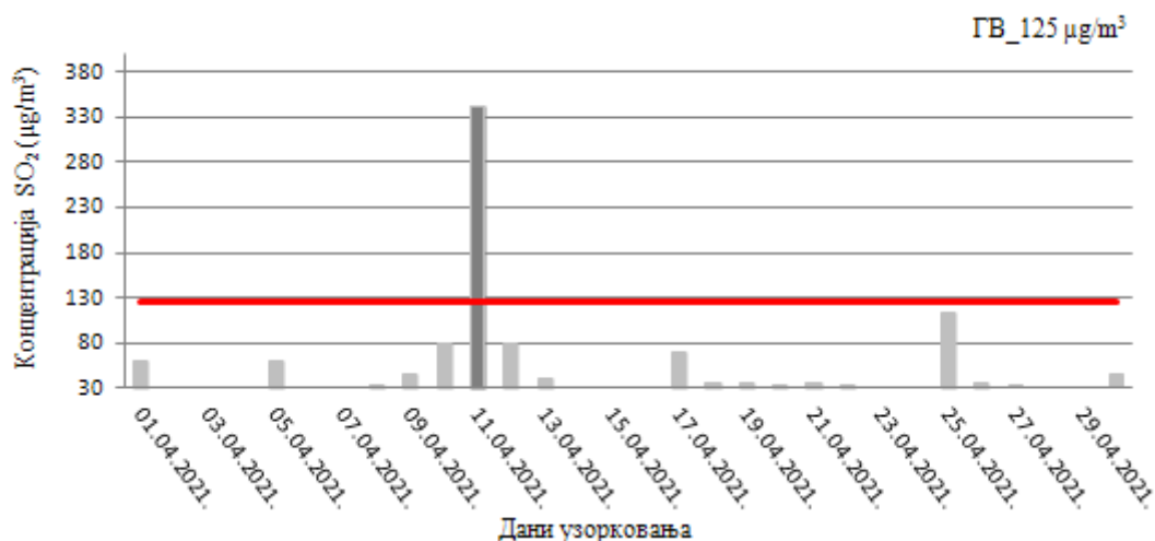
Слика 25. Резултати концентрације SO_2 у ваздуху, на мерном месту 44899-21_F_Технички факултет
